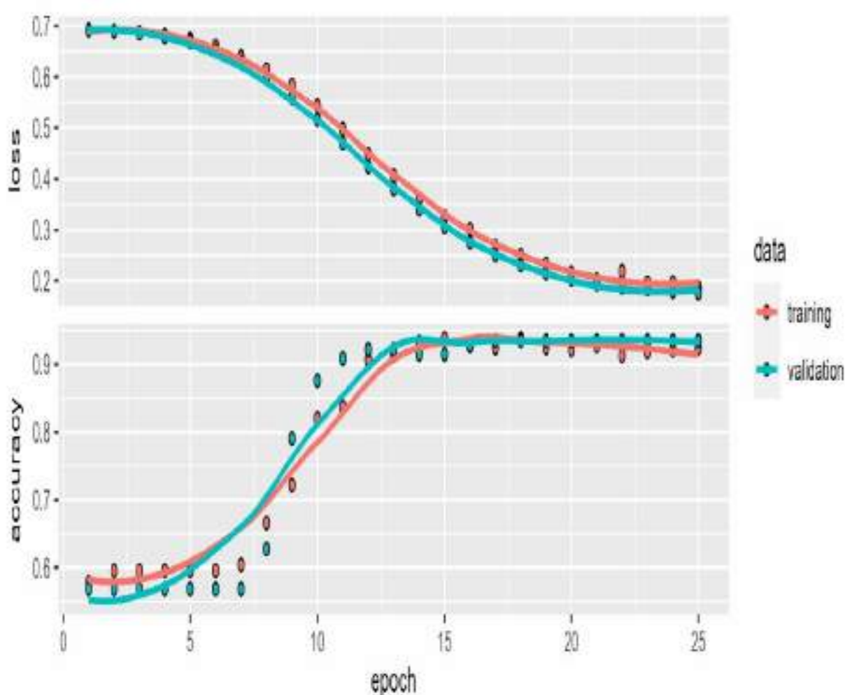
Рисунок 7.1 – Навчання нейронної мережі для прогнозування рівня теплочутливості на основі психофізіологічних параметрів
